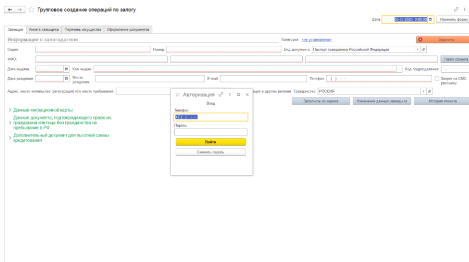
Рисунок 4. Авторизация пользователя
