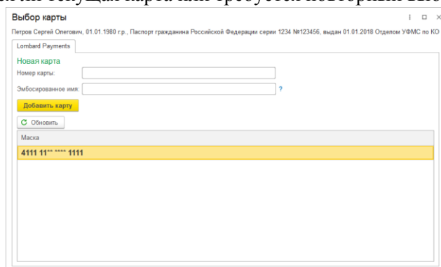
Рисунок 6. Выбор карты
